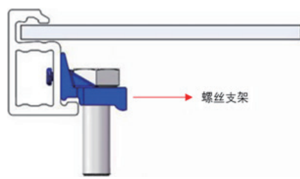
螺丝支架安装方式
