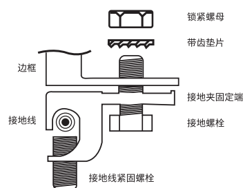
图6 安装方式
