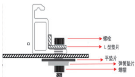
C面开孔安装方式
