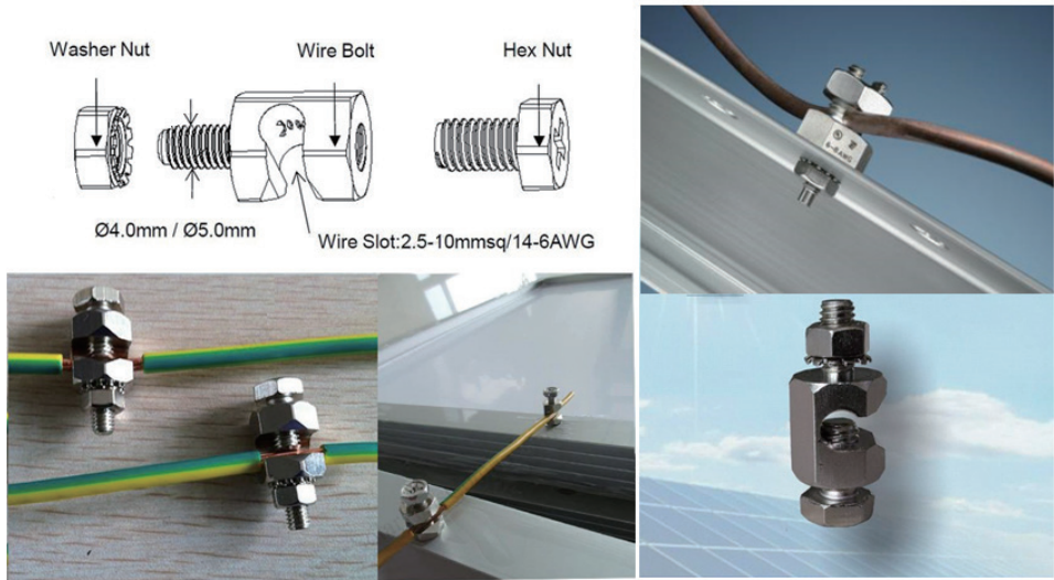
图 5 接地方式
