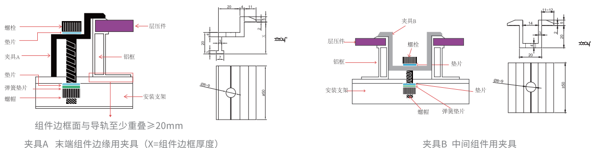
图1 安装夹具细节 (单位: mm)
